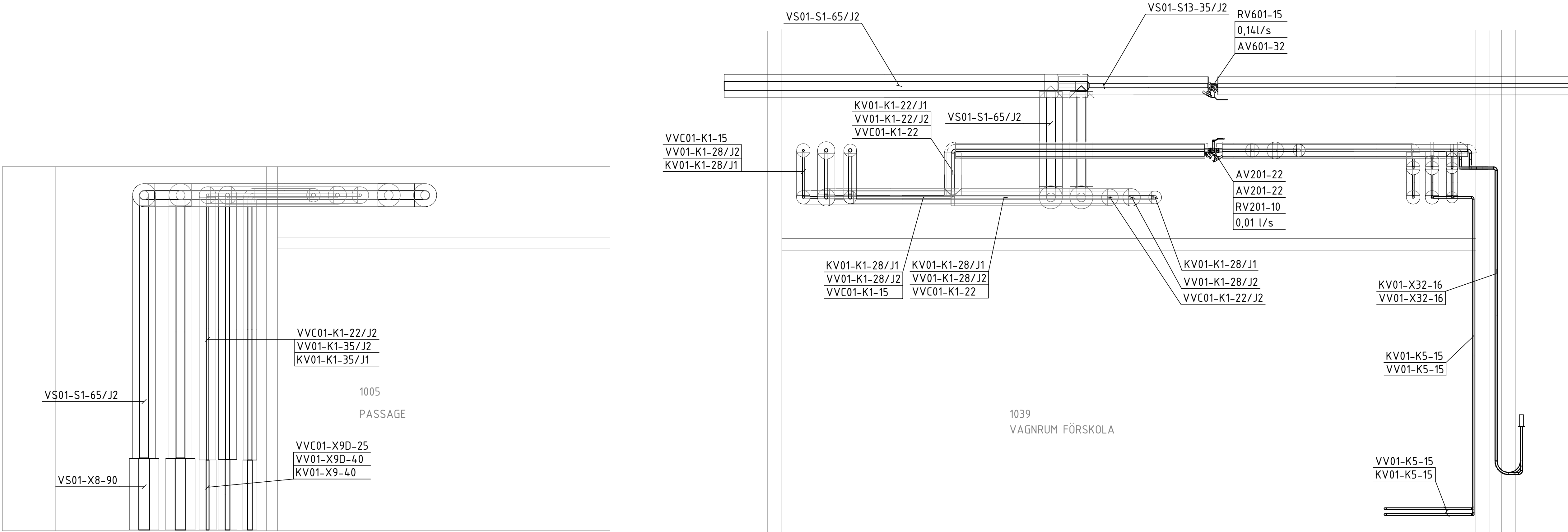
SEKTION 6 SKALA 1:20
