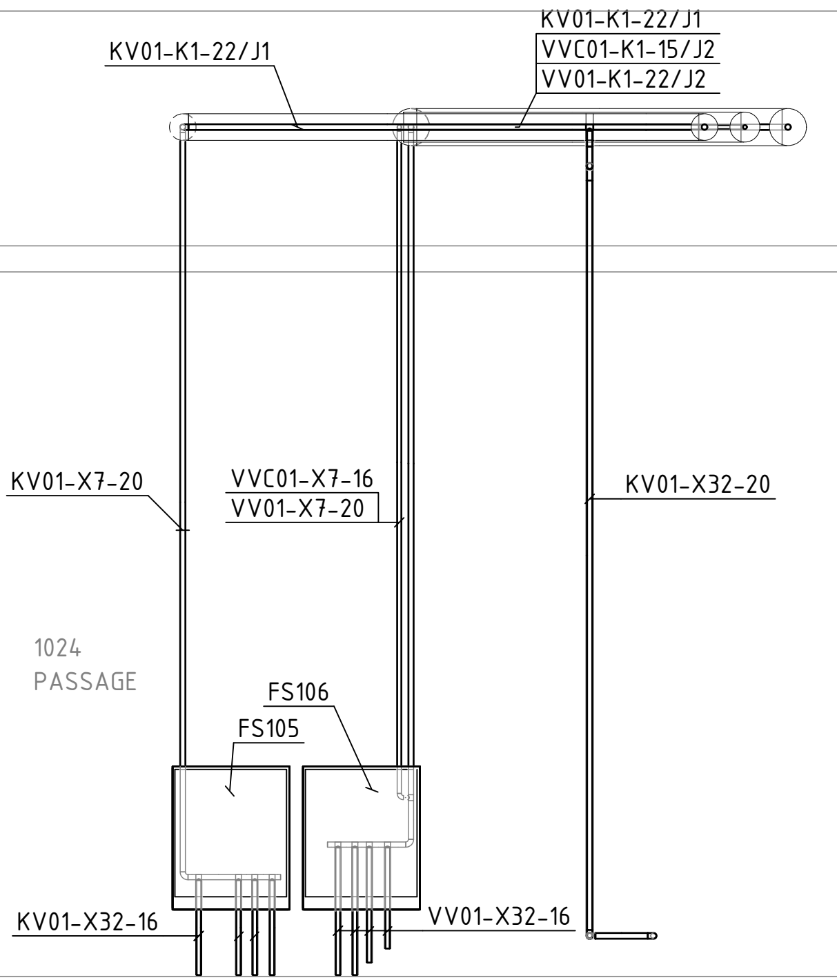
SEKTION 8 SKALA 1:20
