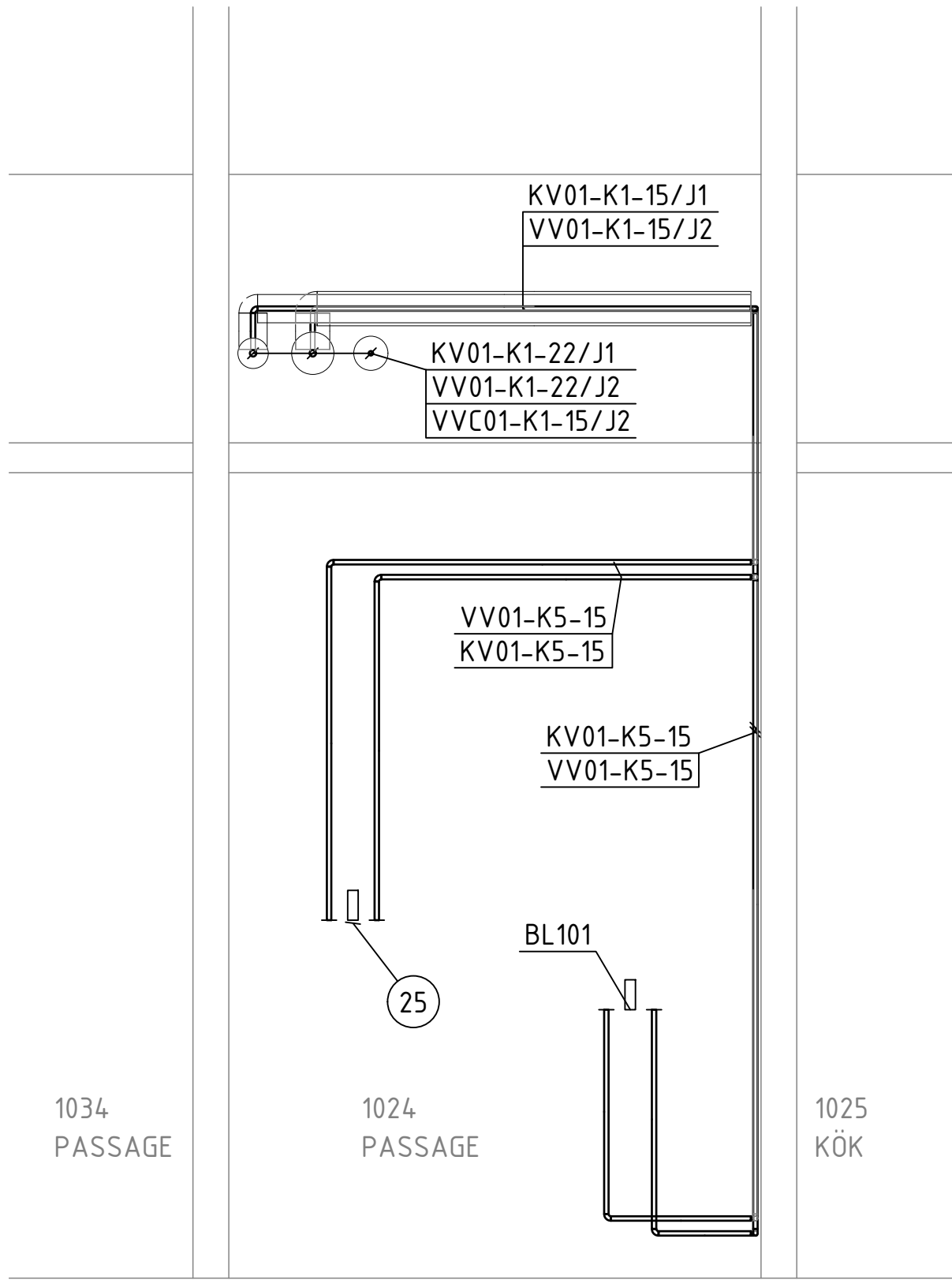
SEKTION 7 SKALA 1:20
